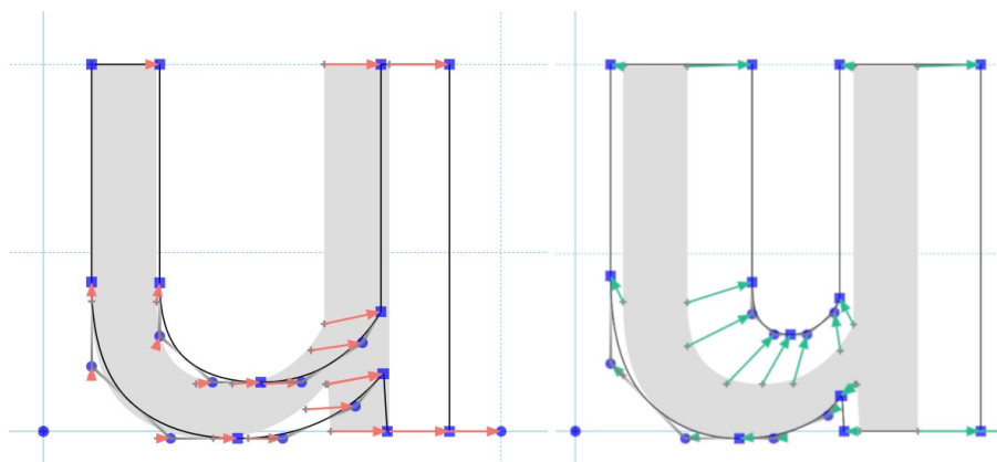
FIGURE 5 – Masters (ici le minimal est en gris, le maximal dessiné par contours) et vecteurs définissant les variations du « u » d'une fonte selon l'axe width (à gauche) ou weight (à droite).
